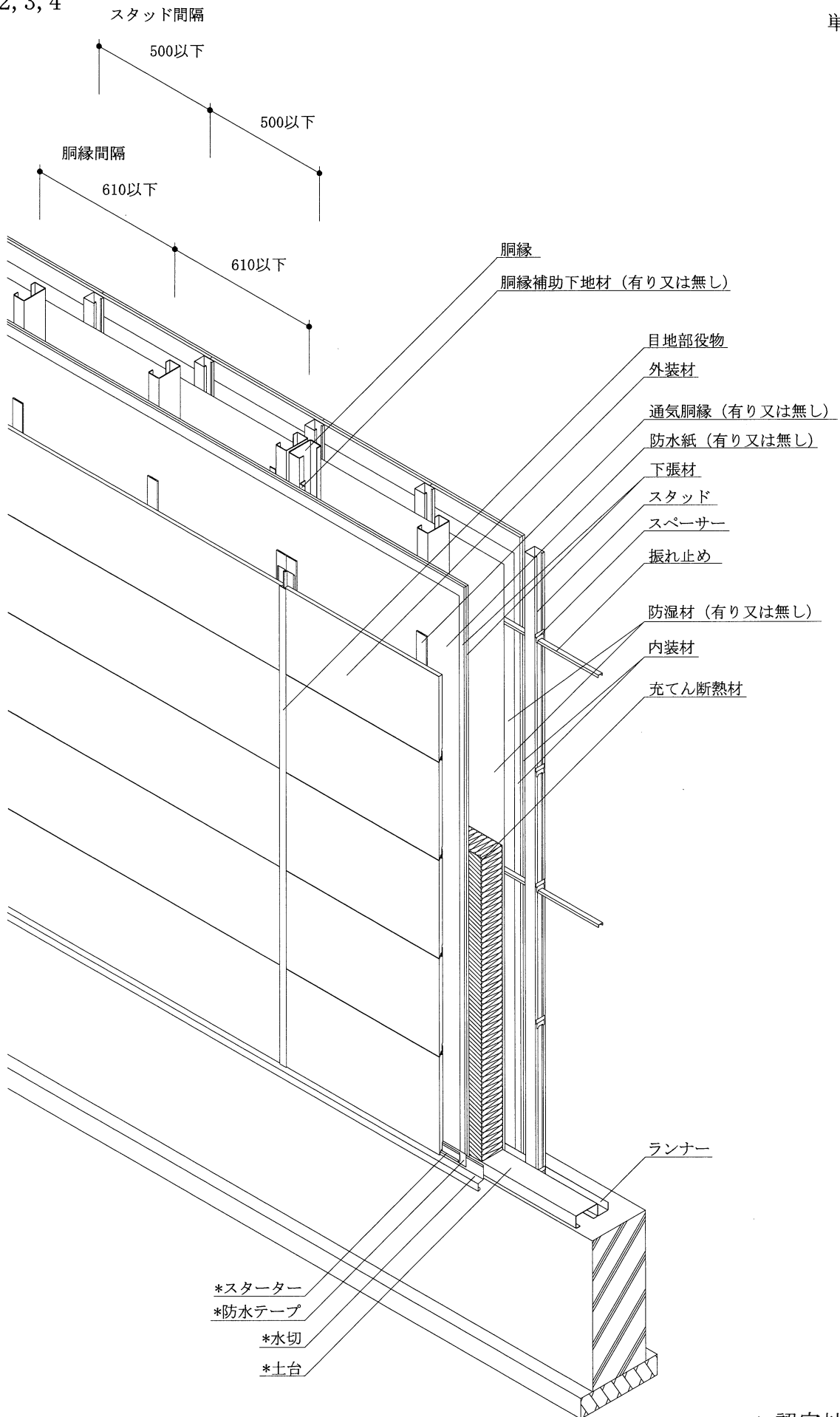
透視図 (別添-15)
