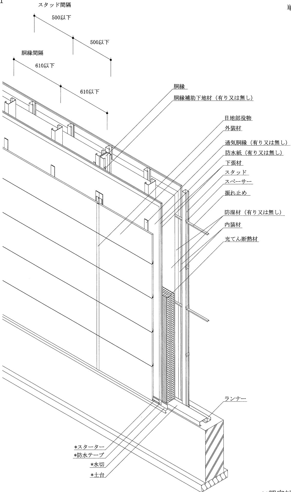
透視図 (別添-14)
